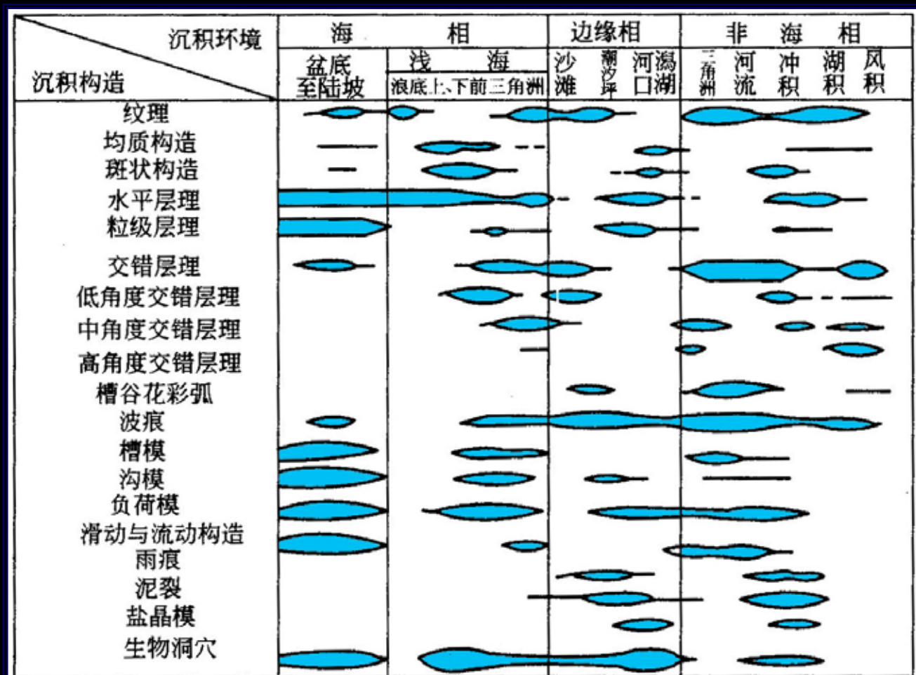
主要沉积环境中各种沉积构造的分布 (据 Heckel, 1972)
