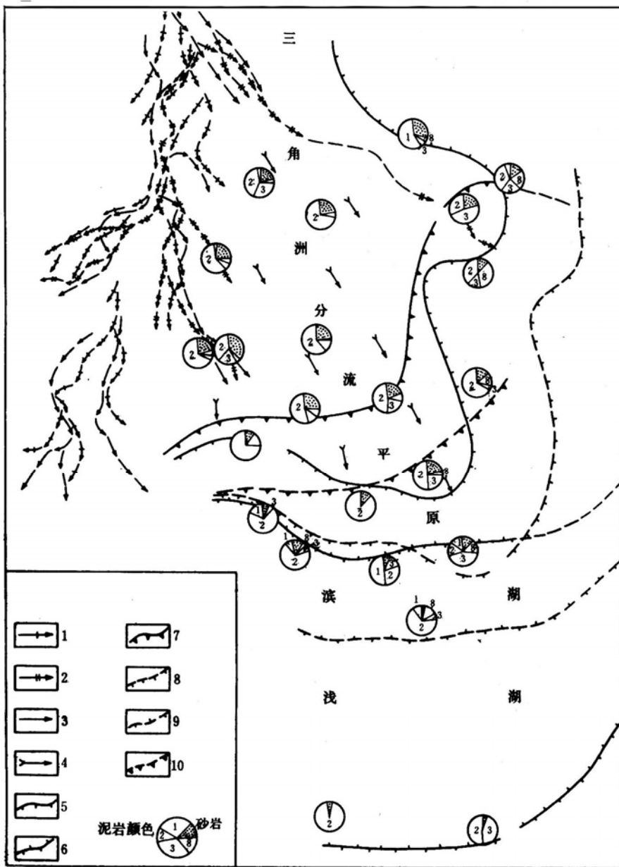
松辽盆地三肇地区姚一段水体系图
