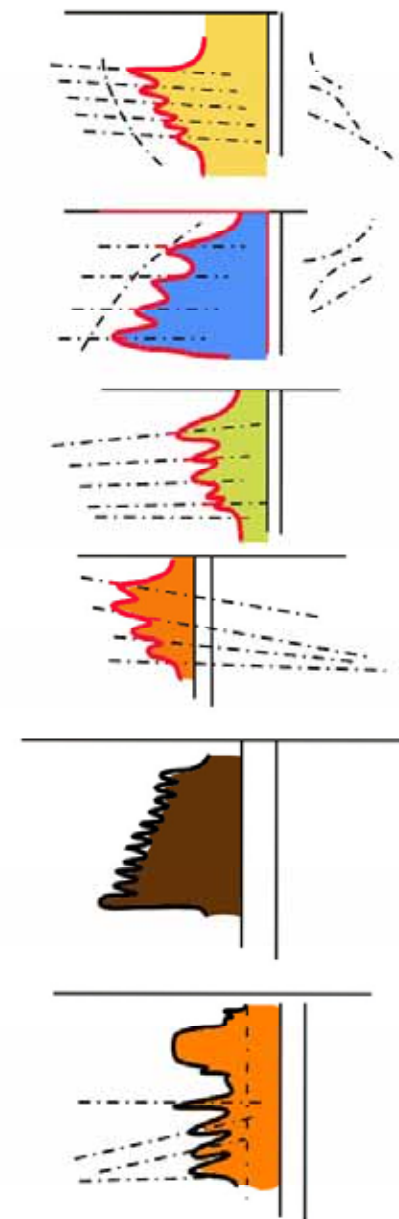
根据自然电位曲线划分的主要沉积层序 (a)水退；(b)水进；(c)岸外砂坝； (d)河道充填砂坝；(e)浊流；(f)三角洲
