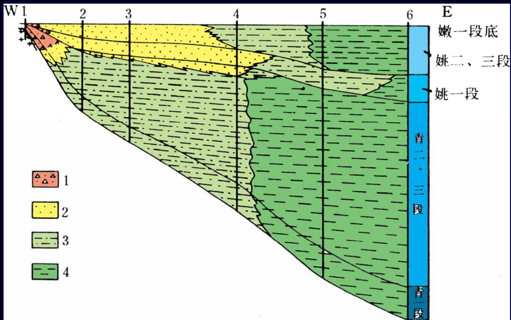
松辽盆地白垩系英台沉积体系岩相剖面图
